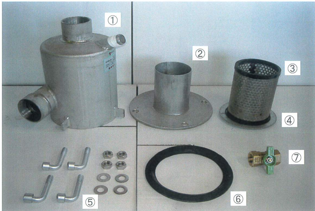
③フィルター部 ④逆流防止円盤
